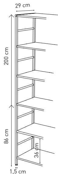
SPALLE Prof. 29 cm UPRIGHTS Depth 29 cm
