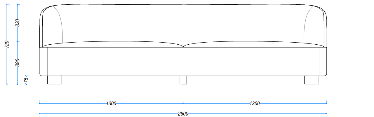
PROSPETTO FRONTALE
