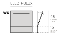
Dishwasher with Fantin door Lavastoviglie con anta Fantin Geschirrspüler mit Fantin Tür
