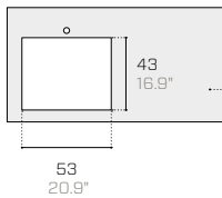
Hole size for the S1 sink Foratura top per vasca S1 Größe der Bohrungen für Beck S1
