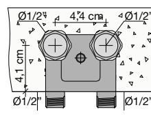
Allacciamento del TBT
