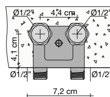
Allacciamento del TBT
