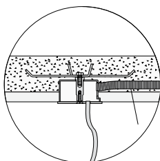
Particolare "B" Per soletta in CEMENTO
