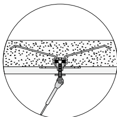
Particolare "B" Per struttura in LATERIZIO
