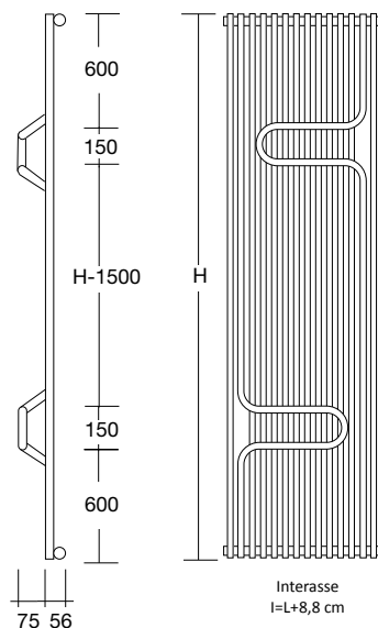
AK2 - VERSIONE IDRAULICA STANDARD DOPPIO MANIGLIONE (Attacchi OC1)
