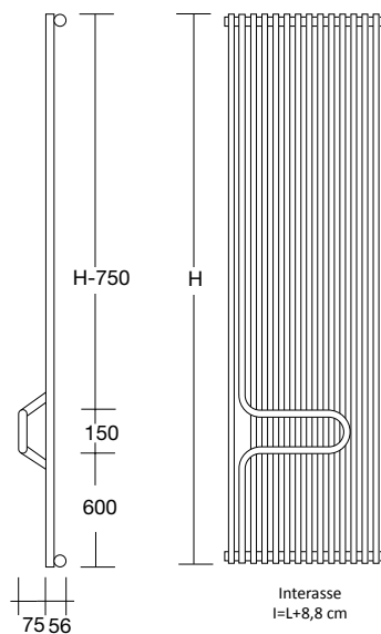
AK - VERSIONE IDRAULICA STANDARD (Attacchi OC1)
